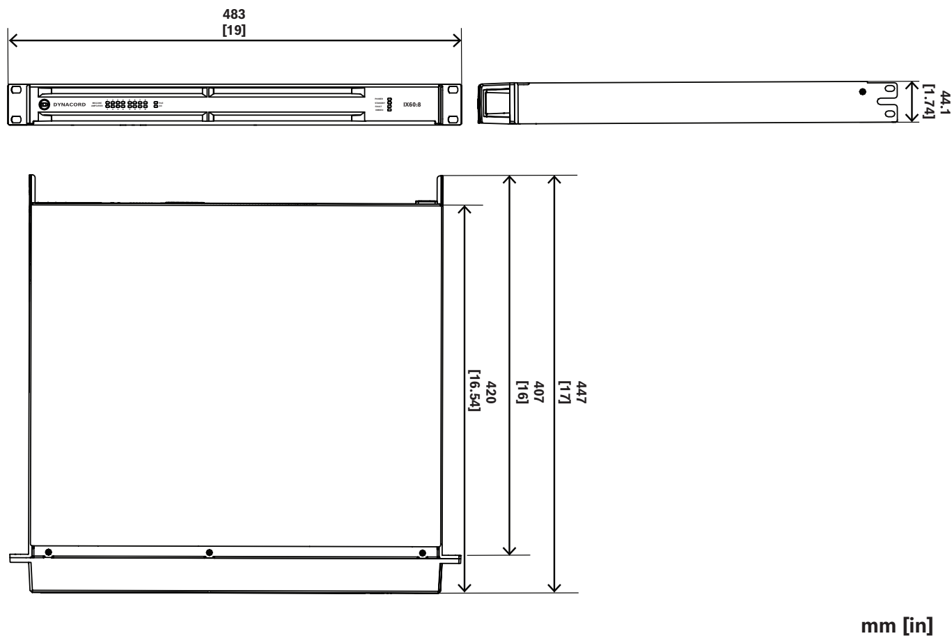
Fig. 4: Dimensions
