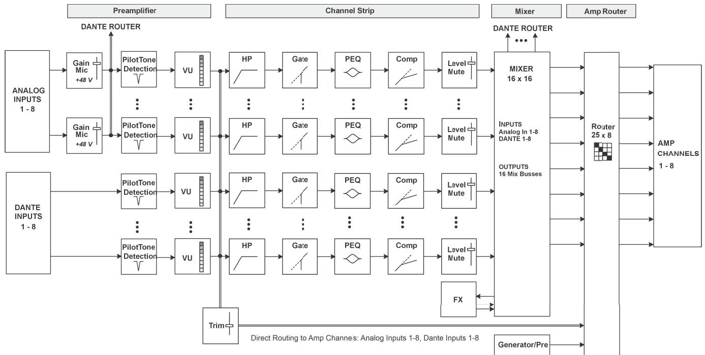
Abb. 1: Eingangsblockdiagramm
