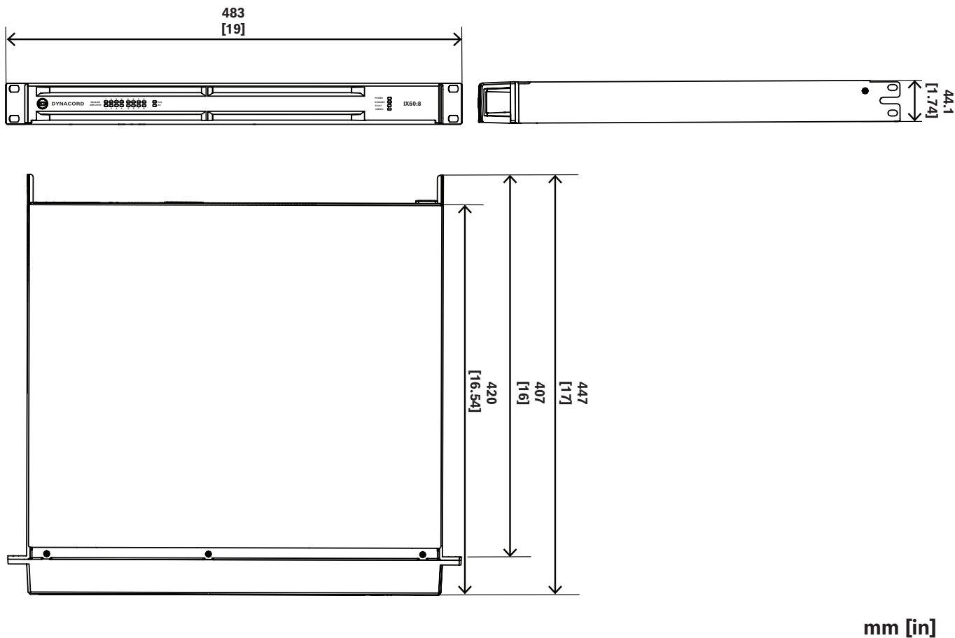
Abb. 4: Maße
