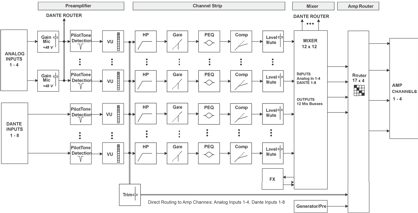
Abb. 1: Eingangsblockdiagramm
