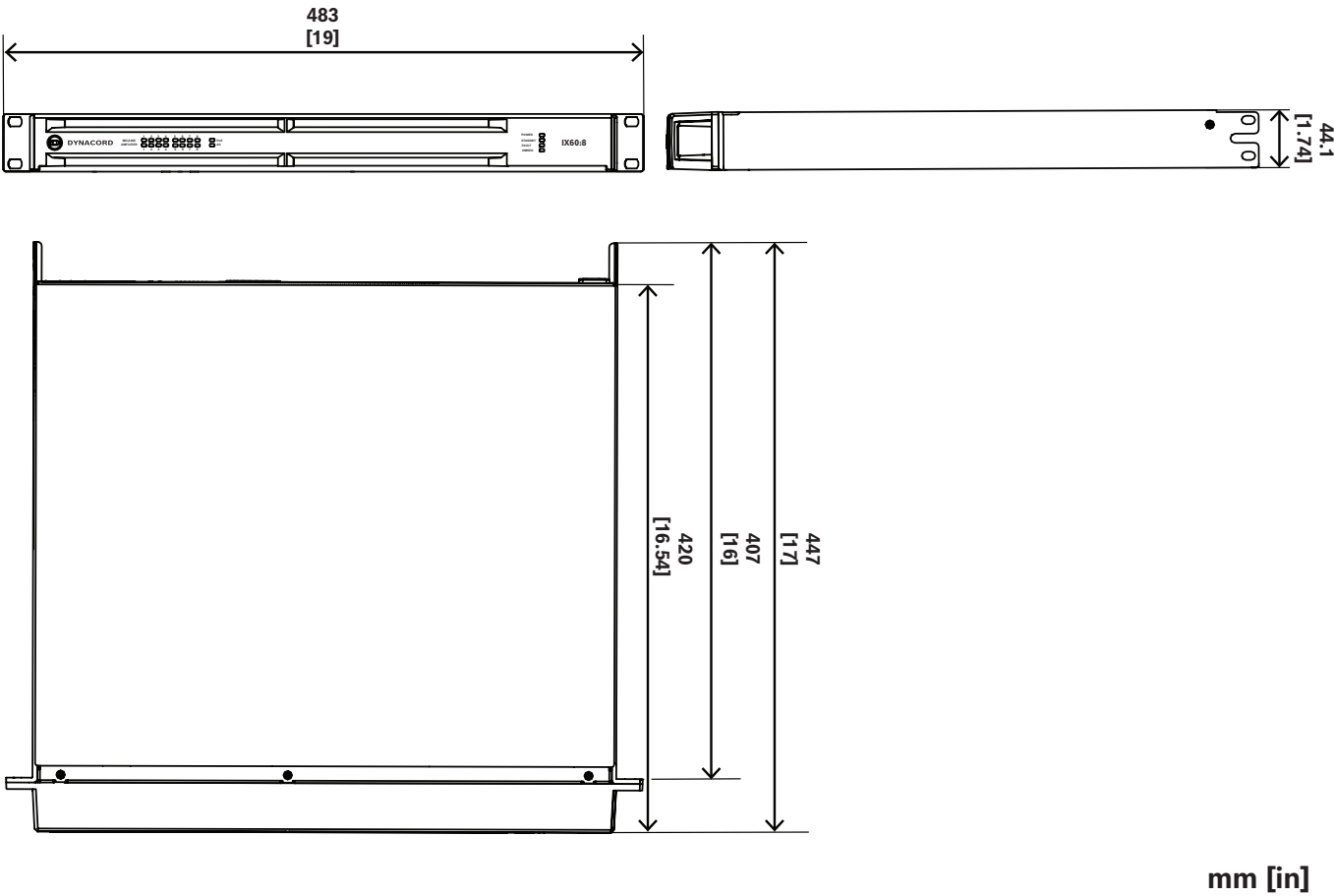
Fig. 4: Dimensions
