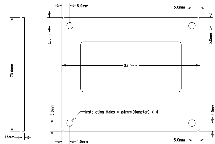
Abbildung 10.2: Abmessungen der LCD-Platine
