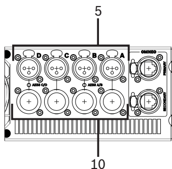
図 6.3: TGX 音声コネクタ
