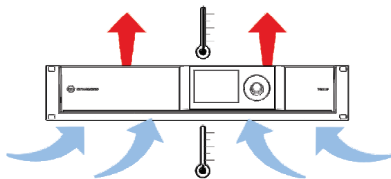
図 5.1: パワーアンプの通気
