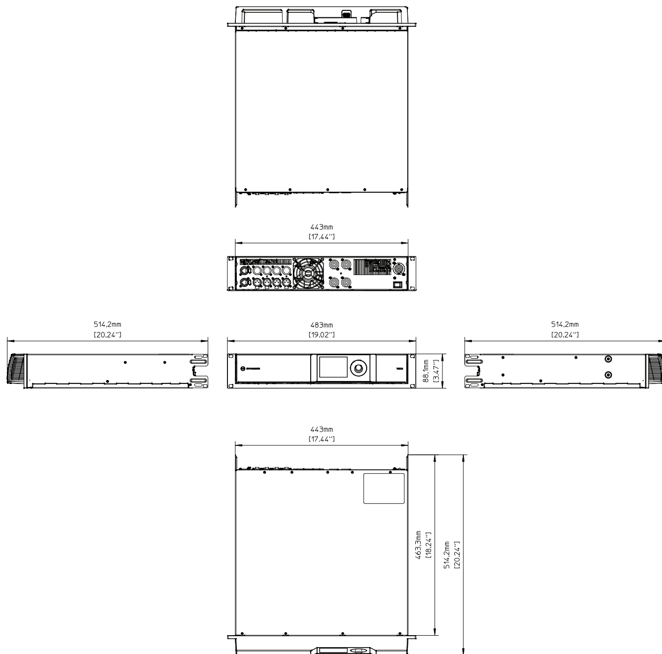
図 8.2: 寸法 : TGX
