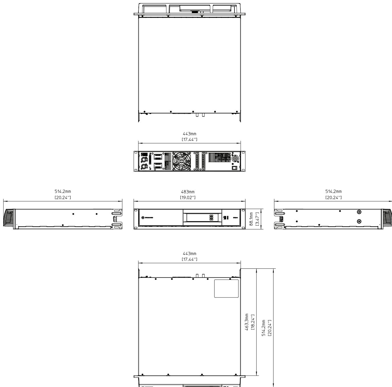
Fig. 2: Dimensioni: IPX
