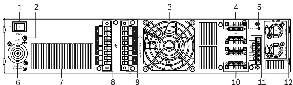
Figura 6.2: Painel traseiro do IPX
