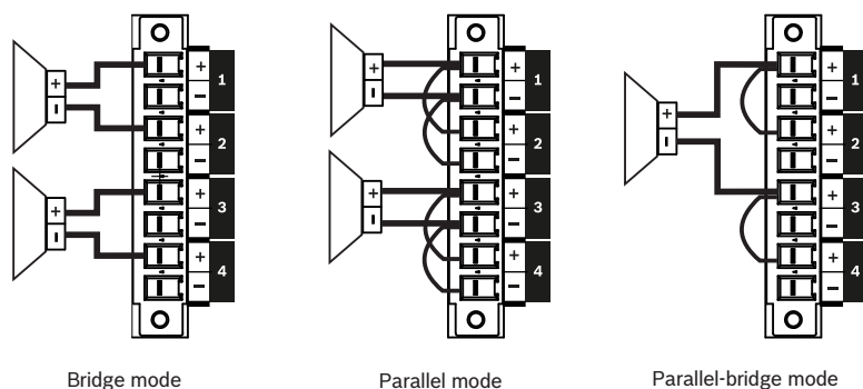
Figura 6.5: Cabos de saída para modos de operação diferentes nos amplificadores que combinam 2 ou 4 canais.
