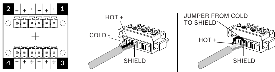
Figura 6.6: Conectores de entrada, fiação para operação balanceada, fiação para operação não balanceada
