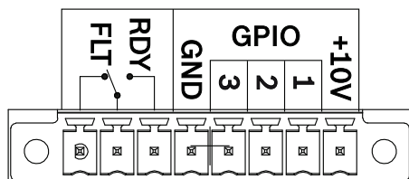
Figura 6.3: Porta de controle
