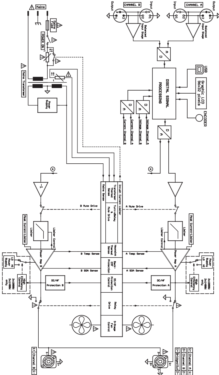
그림 2: 블록 다이어그램
