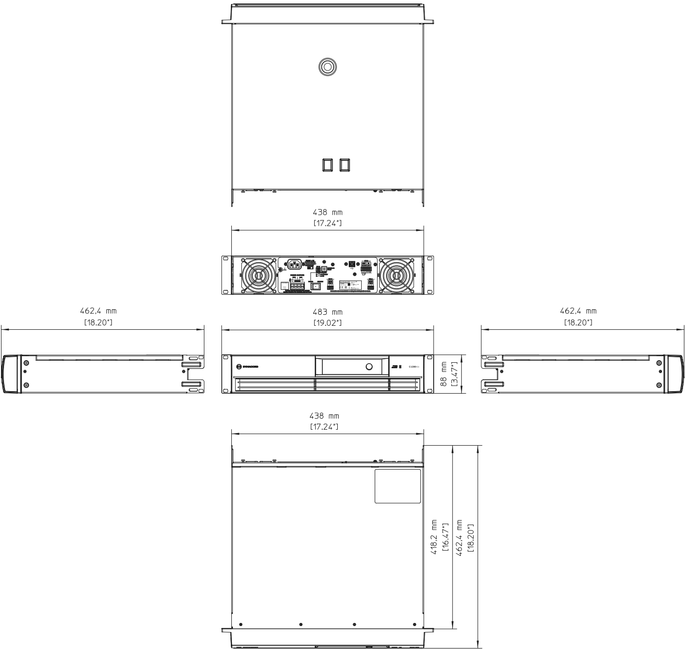
Fig. 1: Dimensioni
