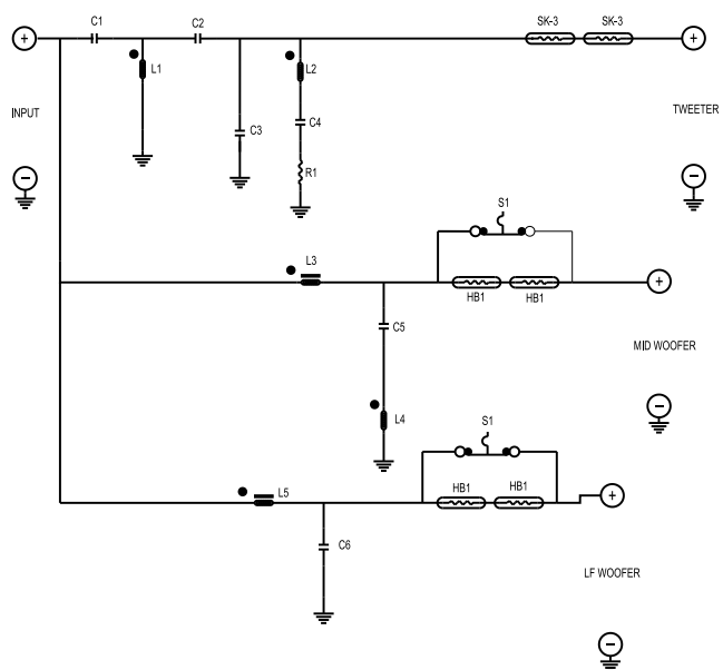
회로도
