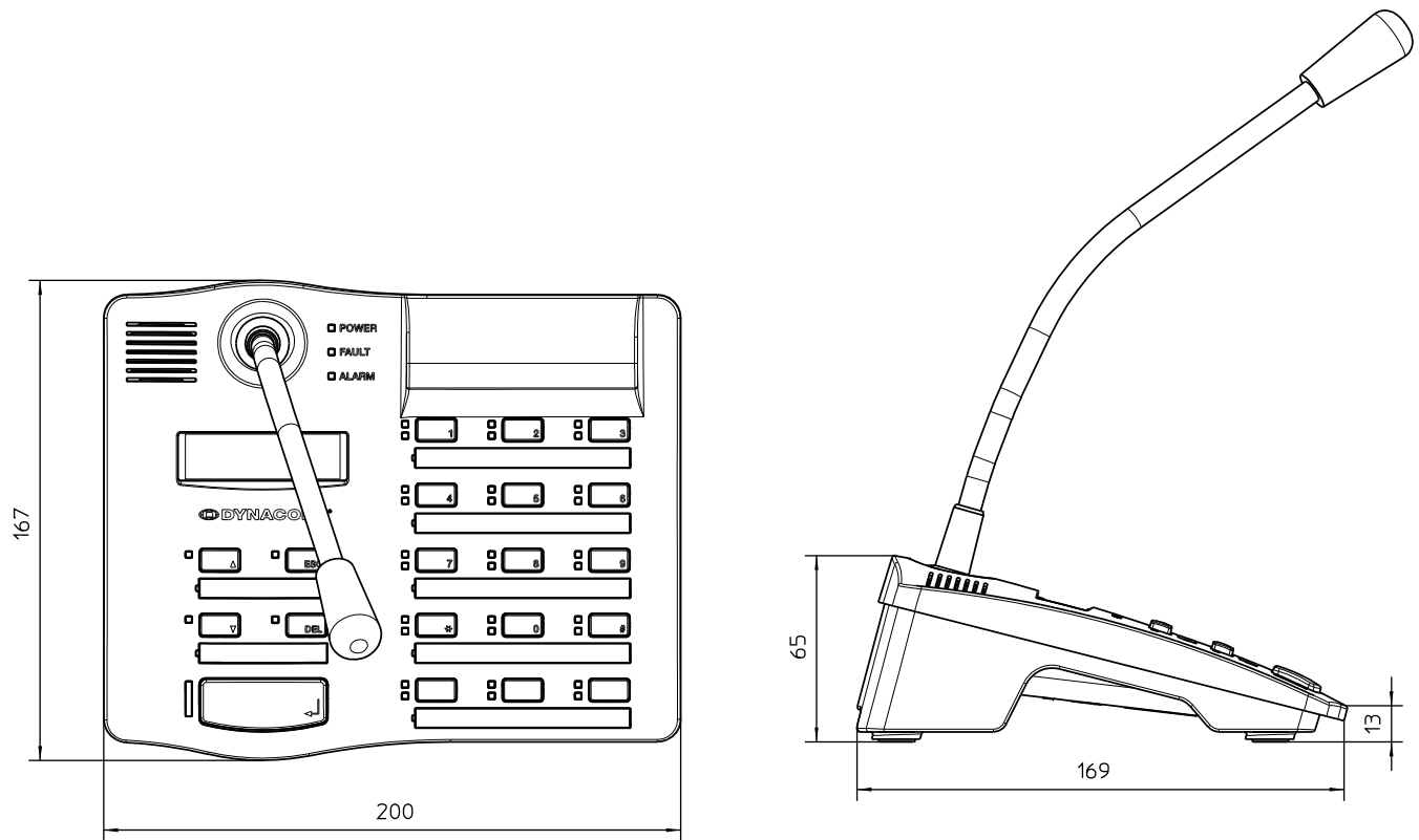
Figure 10.1: DPC 8015
